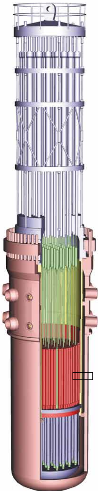
A reaktortartály a felügyeleti próbatetekkel
